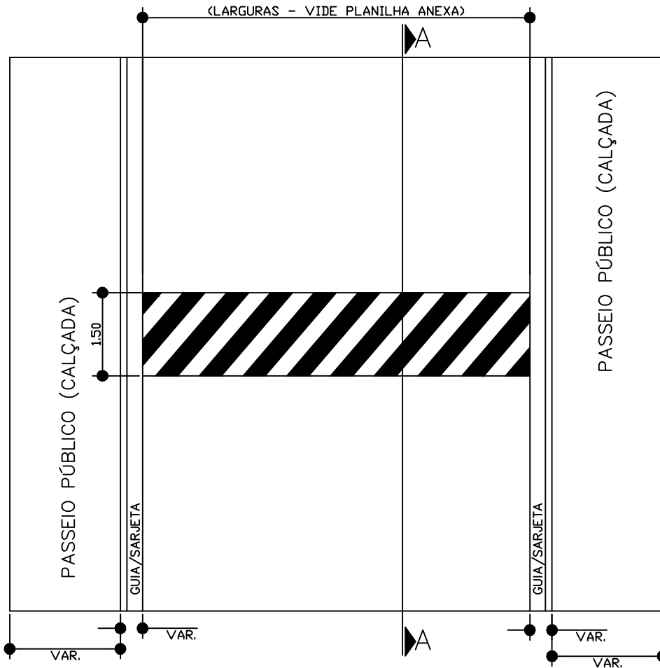
PLANTA BAIXA 1:100
