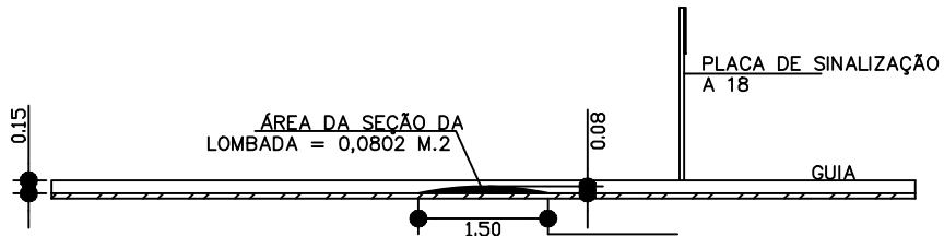
CORTE AA 1:100
